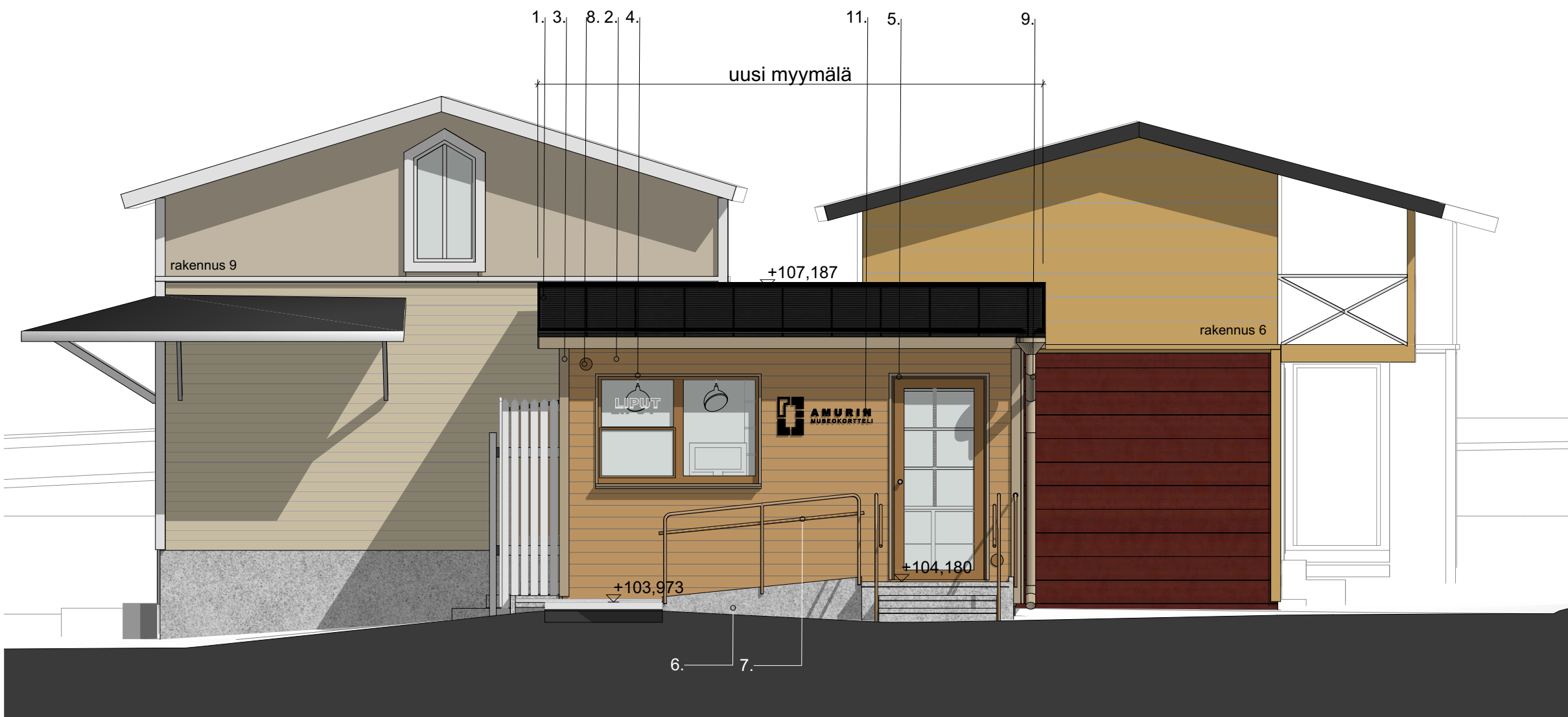
Julkisivu pohjoiseen 1:50
