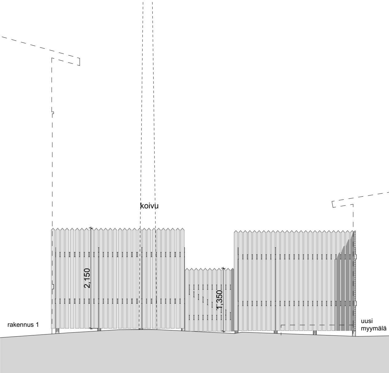
aita Projektio 1:50
